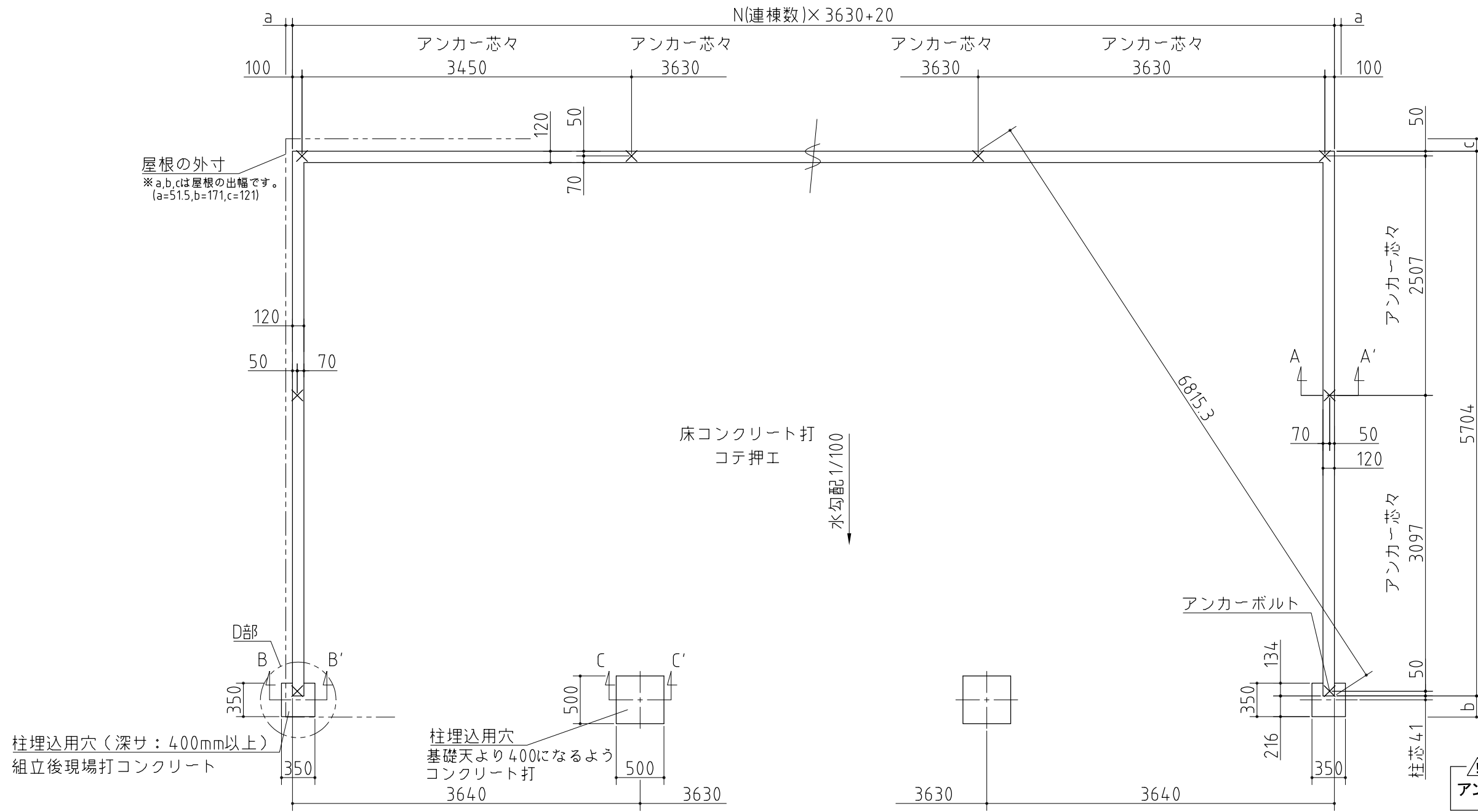
基礎詳細図 S=1/20
